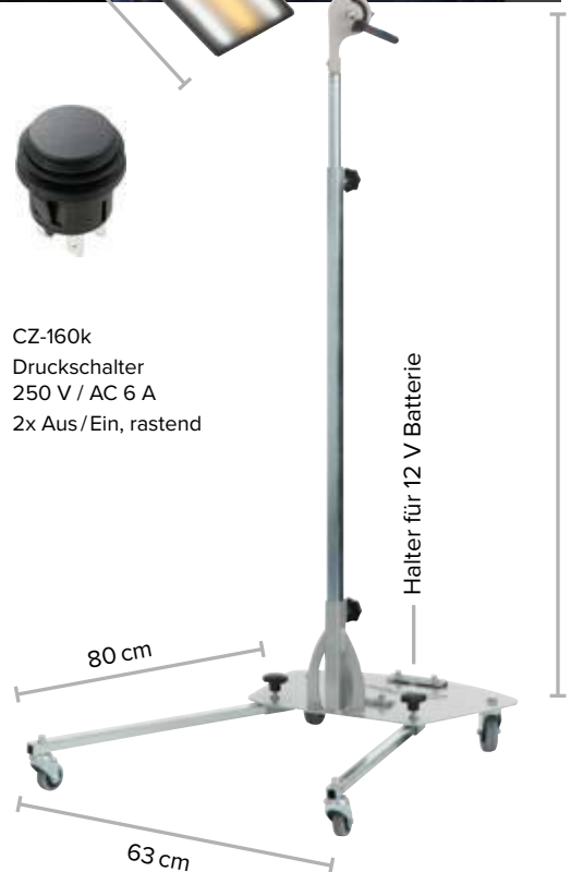
CZ-160 Moderne, energiesparende LED-Leuchte für Normal- und Schattenlicht. Der Lam- penkörper ist variabel höhenverstellbar und 360° drehbar
